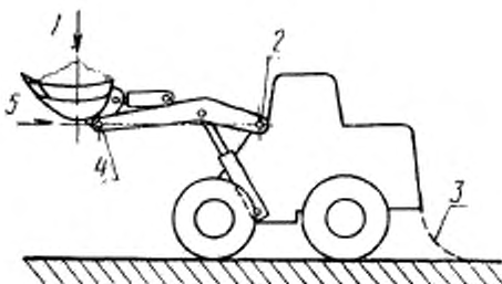
Типовая схема испытаний по определению максимальной опрокидывающей нагрузки на максимальном вылете
