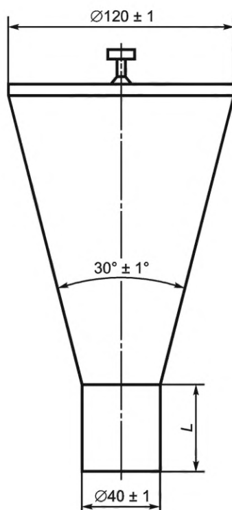
Рисунок 14 — Испытательный конус
