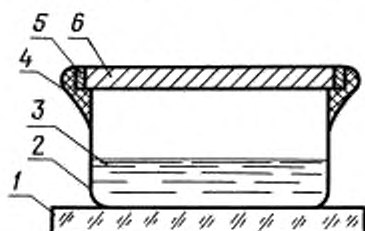
Схема прибора для определения сопротивления паропроницаемости
