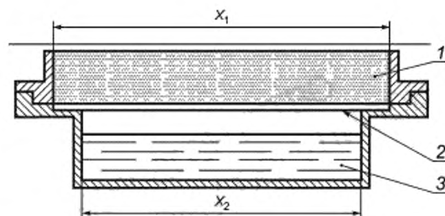
1 — испытуемый образец сыпучего материала; 2 — решетка или паропроницаемая мембрана; 3 — дистиллированная вода
