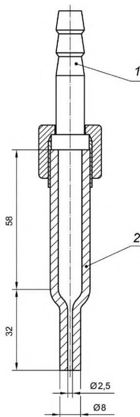
1 — соединительная трубка; 2 — пробоотборная трубка
