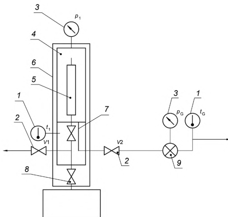
1 — датчик измерения температуры ( t_1 , t_G ); 2 — клапаны сброса давления ( V1 , V2 ); 3 — датчики давления ( p_1 , p_G ); 4 — камера для отбора проб при высоком давлении (см. рисунок 2); 5 — пробоотборная трубка; 6 — теплоизоляция; 7 — клапан камеры; 8 — пробоотборный клапан; 9 — газовый счетчик
