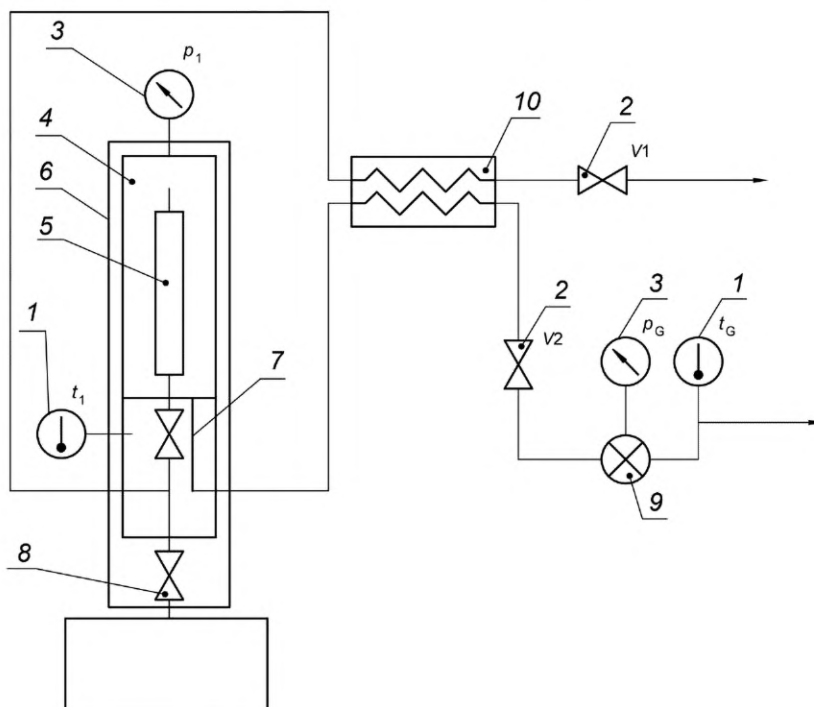
1 — датчик измерения температуры ( t_1 , t_G ); 2 — клапаны сброса давления ( V1 , V2 ); 3 — датчики давления ( p_1 , p_G ); 4 — камера для отбора проб при высоком давлении; 5 — пробоотборная трубка; 6 — теплоизоляция; 7 — клапан камеры; 8 — пробоотборный клапан; 9 — газовый счетчик; 10 — теплообменник
