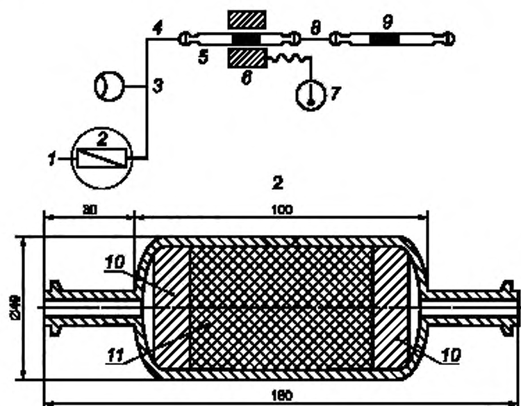
1 — воздушный насос; 2 — ловушка для ртути; 3 — ротаметр; 4 — трубки из ПВА; 5 — пробоотборная трубка; 6 — печь для трубок; 7 — термометр; 8 — соединительная стеклянная трубка; 9 — аналитическая трубка; 10 — стекловолно; 11 — адсорбент (например, активированный уголь, обработанный серой)
