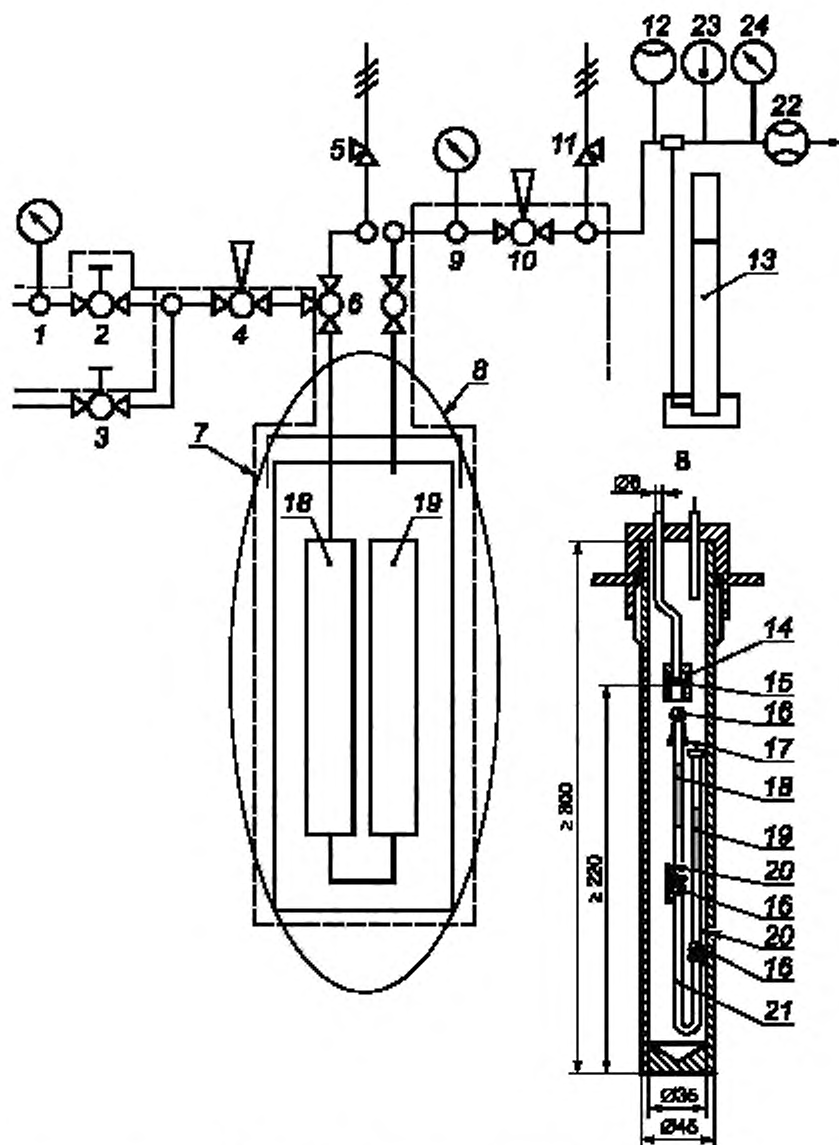
1 — средство измерений давления (от 0 до 25 МПа); 2 — вентиль; 3 — вентиль байпасной линии; 4 — редуктор; 5 — клапан сброса давления, установленный на 10 МПа; 6 — трехходовой кран; 7 — нагревательная лента; 8 — сосуд высокого давления; 9 — средство измерений давления (от 0 до 10 МПа); 10 — редуктор; 11 — клапан сброса давления, установленный на 4 кПа; 12 — указатель расхода (ротаметр); 13 — водяной затвор со столбом воды высотой 0,4 м; 14 — фиксатор с резьбой М20; 15 — шаровидная муфта; 16 — уплотнительное кольцо; 17 — съемный винт (политетрафторэтилен) с резьбой М20; 18 — первая пробоотборная трубка; 19 — вторая пробоотборная трубка; 20 — хомут; 21 — фитинг; 22 — средство измерений объема газа; 23 — средство измерений температуры; 24 — средство измерений давления (от 0 до 16 кПа)
