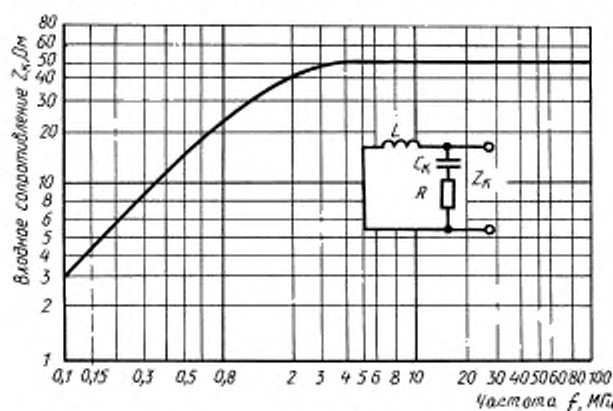
C_k — емкость; R — сопротивление; L — индуктивность
