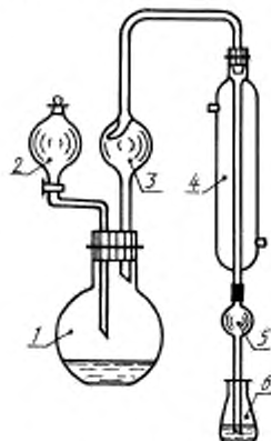
1 — круглая плоскодонная колба вместимостью 1 дм 3 ; 2 — капельная воронка вместимостью 100 см 3 ; 3 — каплеуловитель (насадка Кельдаля); 4 — холодильник с прямой трубкой; 5 — стеклянная трубка длиной 200 мм с шариковым расширением; 6 — колба-приемник вместимостью 250 см 3
