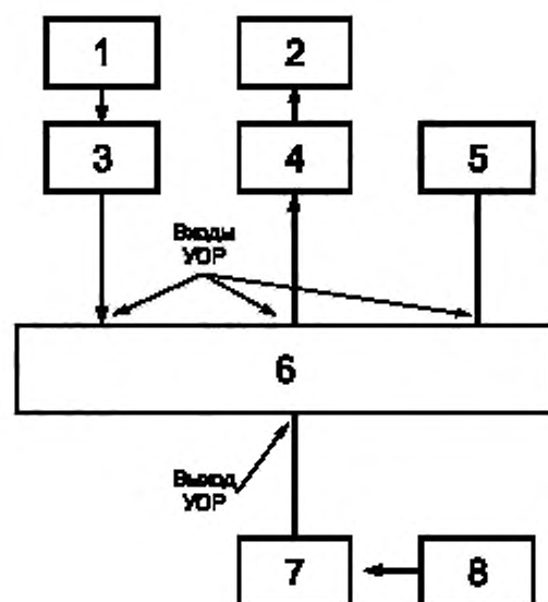
1 — генератор сигналов ВЧ; 2 — селективный микрольтметр; 3, 4 — согласованные коаксиальные переходы; 6 — УОР; 5, 7 — согласованные экранированные нагрузки; 8 — милливольтметр ВЧ
