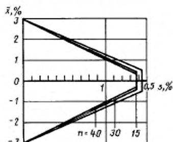
Метод \bar{x}, s
