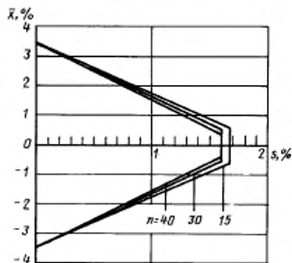
Метод \bar{x}, s
