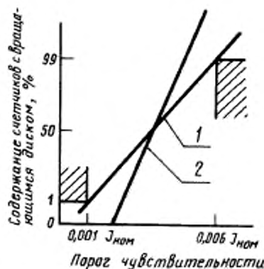
1 — распределение в наиболее неблагоприятном случае; 2 — распределение, действительное для данной партии
