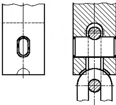
Рисунок 5 — Обойма захватов
