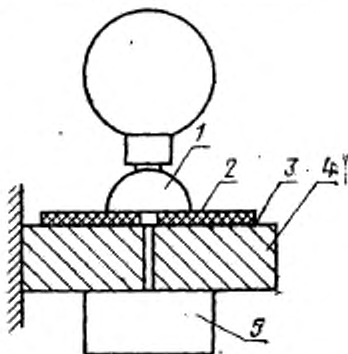
1 — испытательный электрод; 2 — уплотнительный лист (например из мягкой резины, ориентировочные размеры: 3 \times 50 \times 50 мм); 3 — слой клея; 4 — основной материал; 5 — вакуумметр
