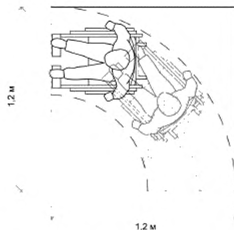
Рисунок Б.2 — Пространство для поворота на 90^\circ
