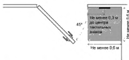
Рисунок 11 — Размещение информации при угловом расположении двери на расстоянии более 0,6 м от боковой стены
