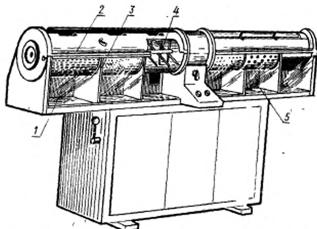
1 — рабочая камера; 2 — загрузочная воронка; 3 — перегородка; 4 — вал с колками; 5 — сетка
