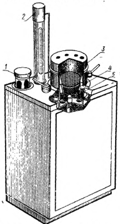
1 — регулятор уровня; 2 — ротаметр; 3 — сетка № 1 или 0,5; 4 — сетка № 014; 5 — резиновая диафрагма Черт. 2
