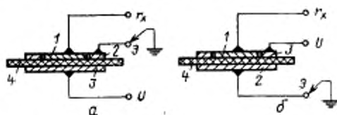
Схема включения электродов в измерительную цепь при измерении объемного R_v (а) и поверхностного R_x (б) сопротивлений
