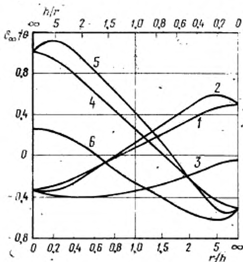
Зависимость отношения \delta_{\infty}/\theta от формы цилиндрического детектора радиуса r и полувысоты h для случаев 1-6 таблицы приложения 6
