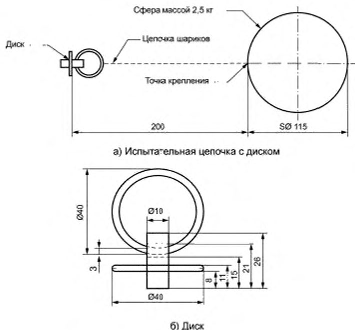
Рисунок 6 — Испытательная цепочка с диском
