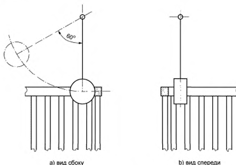
Рисунок 11 — Схема испытания на удар угла кровати
