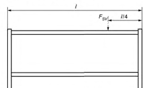
Рисунок 12 — Схема испытания вертикальной статической нагрузкой
