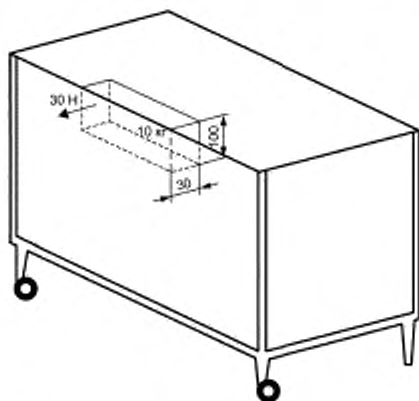
Рисунок 16 — Схема испытания на горизонтальную устойчивость
