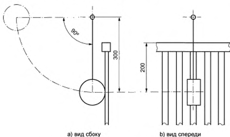
Рисунок 10 — Схема испытания на боковой удар
