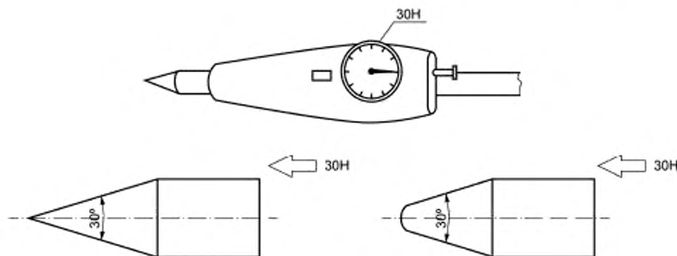
Рисунок 1 — Примеры измерительных конусов
