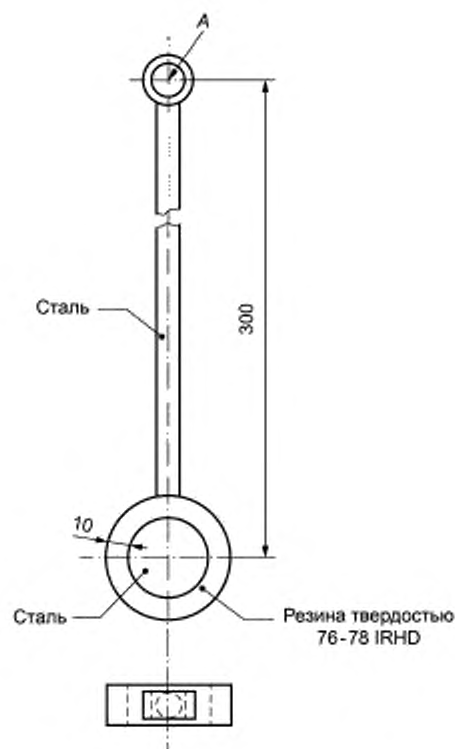
Рисунок 3 — Боковой ударник
