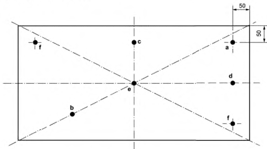
Рисунок 9 — Схема расположения точек ударов
