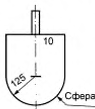
Рисунок 2 — Сбрасываемый ударник
