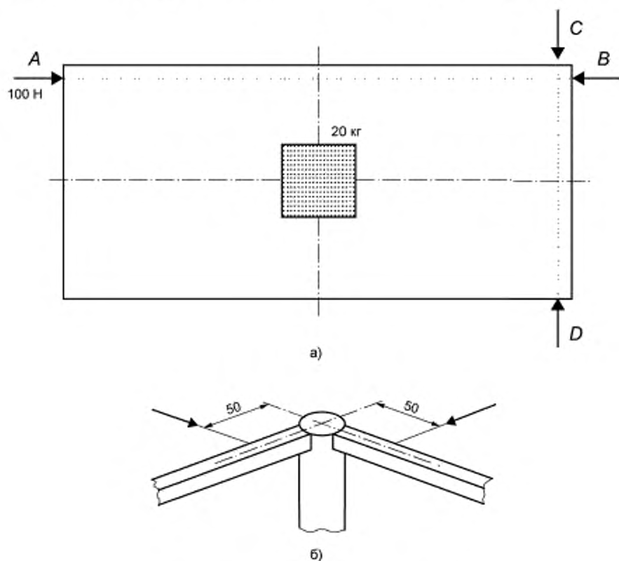
Рисунок 13 — Схема испытания на усталость
