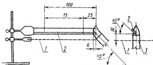
1—металлическая проволочная сетка; 2—испытуемый образец; 3—горелка
