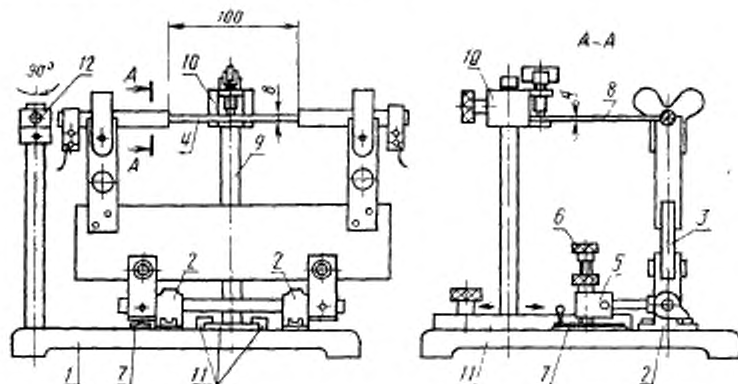
1—плоская плита 2—подшипники; 3—держатель; 4—накаливаемый стержень; 5—противозад. 6—противозад. 7—сопоставитель клапана; 8—испытуемый образец; 9—держатель образца; 10—нагреватель; 11—поднятое основание; 12—поворотный металлический стержень
