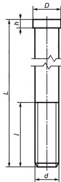
Рисунок 2 — Болт
