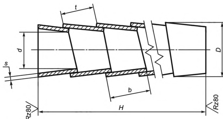
Рисунок 3 — Заклинивающий элемент
