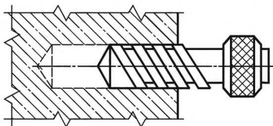
Рисунок 4 — Сверление отверстия
