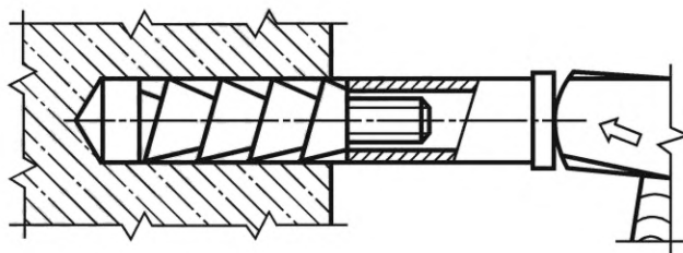
Рисунок 5 — Осаживание заклинивающего элемента
