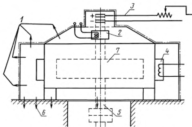
1 — излучение через стенки; 2 — охладитель подшипника; 3 — возбуждение; 4 — основной охладитель; 5 — теплопередача к турбине; 6 — теплопередача к фундаменту; 7 — охлаждающий воздух
