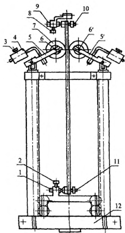
1 — нижний зажим; 2, 8 — затягивающие винты; 3 — закрепляющий винт; 4 — противовес; 5, 5' — нагружающие рычаги; 6, 6' — оси; 7 — ролик; 9 — верхний зажим; 10, 11 — фиксирующие винты; 12 — основание приспособления
