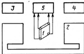
1 — измеряемый образец; 2 — магнит; 3 — источник постоянного тока; 4 — измерительное устройство; 5 — коммутационное устройство
