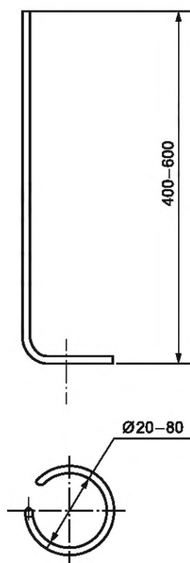
Рисунок 1 — Мешалка
