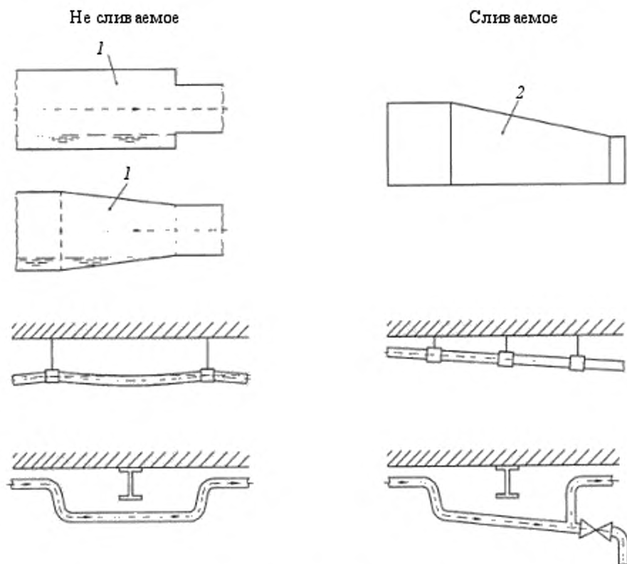
1 – концентричный переходник, 2 – эксцентричный переходник
