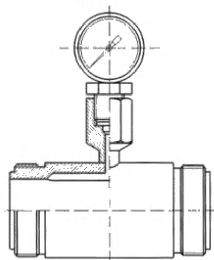
Рисунок А.20 – Приборы (манометры)
