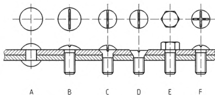
Рисунок А.22 – Крепежные изделия для зоны разбрызгивания
