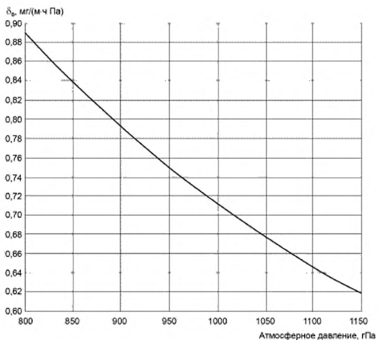
Рисунок Б.1 — Паропроницаемость воздуха при температуре 23 °C
