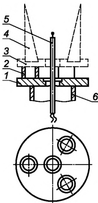
1 — подставка огнеупорная; 2 — опорные кольца; 3 — подставка с испытываемыми конусами; 4 — испытываемые конусы; 5 — термопара; 6 — огнеупорная труба механического приспособления печи
