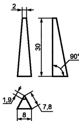
Рисунок 2 — Испытуемый конус
