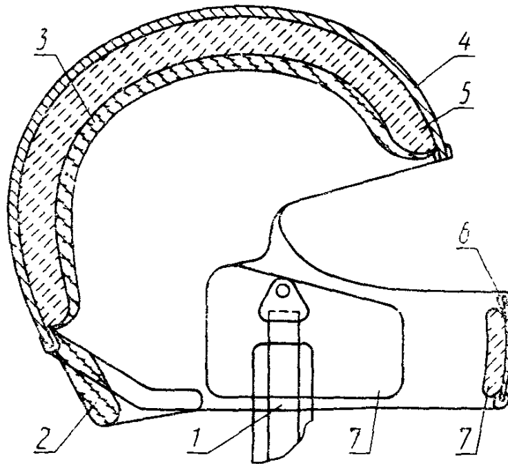
Схема защитного шлема
