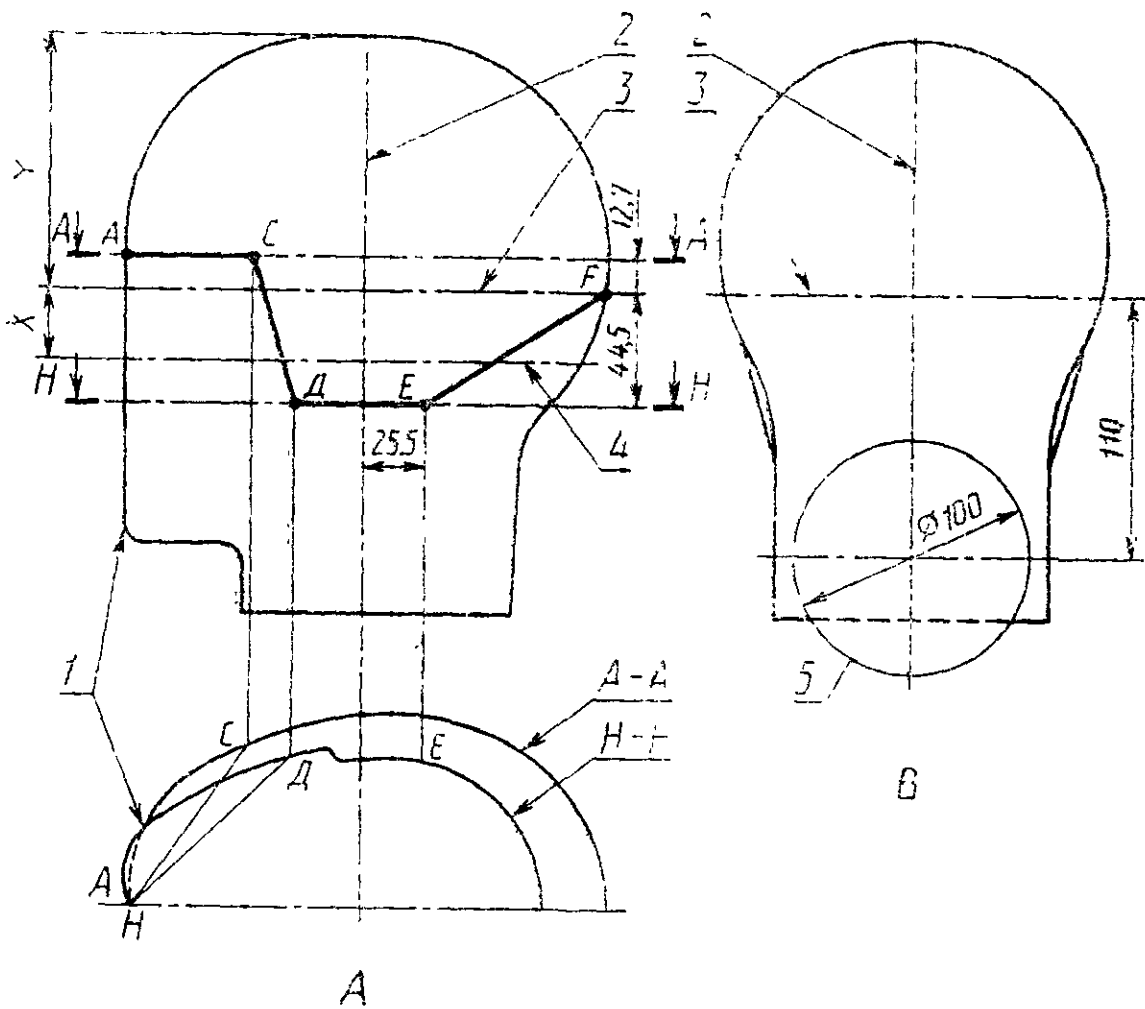
1 — передняя часть муляжа головы, 2 — центральная вертикальная ось, 3 — контрольная плоскость; 4 — основная плоскость, 5 — условный цилиндр
