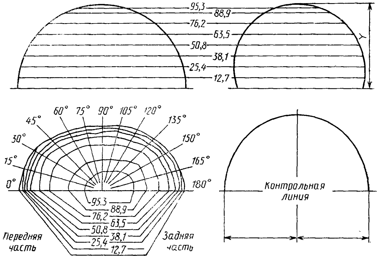
Контрольные муляжи головы (форма и размеры в миллиметрах над контрольной плоскостью)
