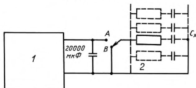
Испытательная схема
