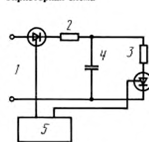
Тиристорная схема
