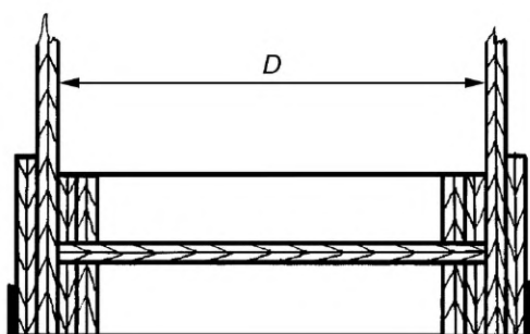
Рисунок А.2 — Крепление фанерного дна к остову фанерными поясками
