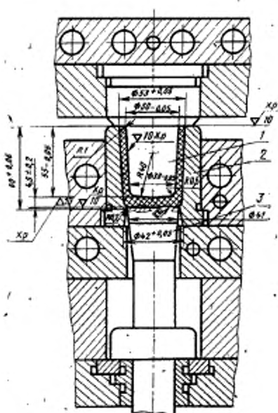
1—пуансон; 2—матрица; 3—выталкиватель.
