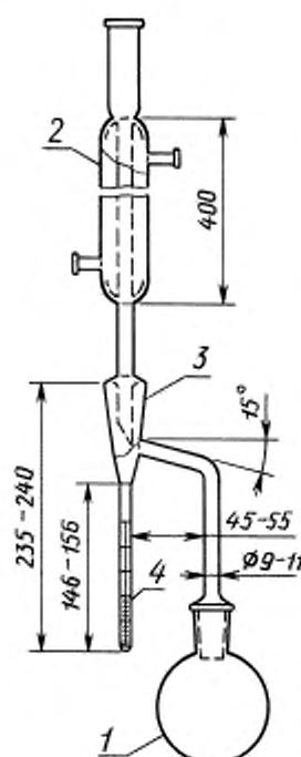
1 — колба; 2 — обратный холодильник; 3 — приемник; 4 — градуированная пробирка
