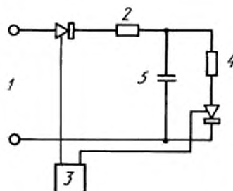
Тиристорная схема
