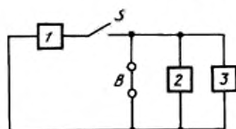
1 — источник постоянного напряжения; S — переключатель; B — перемычка; 2 — измеряемый конденсатор; 3 — запоминающий осциллограф
