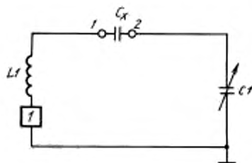
C_x — измеряемый конденсатор; C_I — конденсатор переменной емкости; L_I — индуктивная катушка связи; 1 — индикатор резонанса; 2 — выводы схемы
