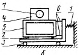
а — схема однокомпонентной установки; б — схема двухкомпонентной установки; 1 — горизонтальные упругие опоры; 2 — вертикальные упругие опоры; 3 — катки; 4 — машина; 5 — опорная плита; 6 — жесткие стержни с шарнирами; 7 — движущаяся часть машины
