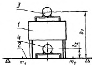
m_1, m_2 — точки, в которых измерялись амплитуды колебаний строительных конструкций; \Delta — опоры строительных конструкций; 1 — машина; 2 — ось строительной конструкции; 3 — первое положение вибратора; 4 — второе положение вибратора
