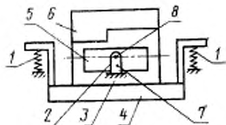
1 — вертикальные упругие опоры; 2 — линейный шарнир; 3 — машина; 4 — опорная плита; 5 — ротор машины; 6 — пригрузка; 7 — центр тяжести машины и опорной плиты (без пригрузки); 8 — центр приложения динамических нагрузок, центр тяжести установки с пригрузкой, центр жесткости упругих опор, ось вращения линейного шарнира
