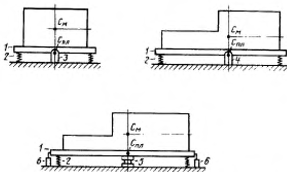
1 — плита стелда; 2 — упругие опоры; 3—5 — съемные линейные шарикоподшипники вдоль осей; 6 — поддерживающие ролики; C_M — центр тяжести машины; C_{пл} — центр тяжести плиты стелда
