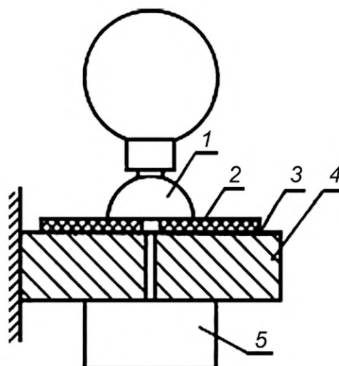
1 — испытуемый электрод; 2 — уплотнительный лист (например, из мягкой резины, ориентировочные размеры: 3 \times 50 \times 50 мм); 3 — слой клея; 4 — основание; 5 — вакуумметр
