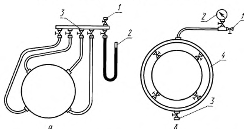
а — отверстия для отбора давления, соединенные с коллектором отдельными трубками; 1 — выпуск воздуха; 2 — жидкостный манометр; 3 — коллектор; б — отверстия для отбора давления, соединенные кольцевым коллектором с манометром; 1 — выпуск воздуха; 2 — манометр; 3 — слив; 4 — кольцевой коллектор
