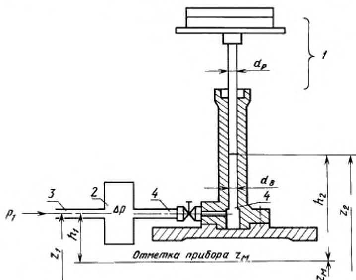
Грузопоршневой манометр, соединенный последовательно с устройством для измерения перепада давлений
