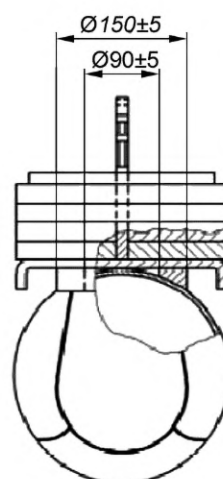
в) Детальный вид удерживающего кольца для мяча
