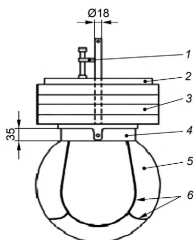
б) Рекомендуемая конструкция
