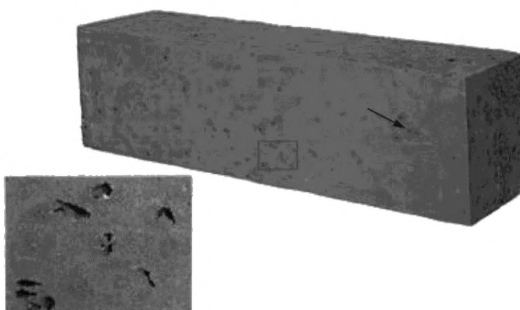
Рисунок А.2 — Выплавка
