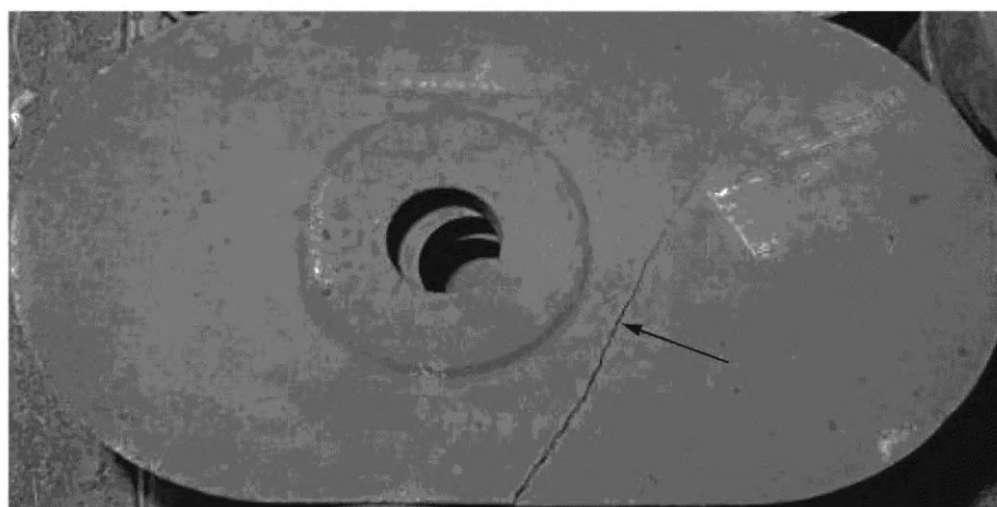
Рисунок А.17 — Трещина
