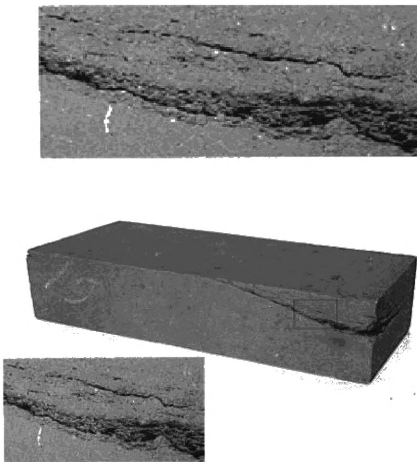
Рисунок А.16 — Слоистость
