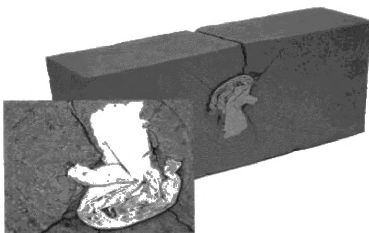
Рисунок А.11 — Постороннее включение
