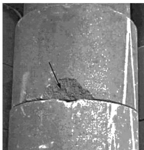
Рисунок А.9 — Отбитость кромки
