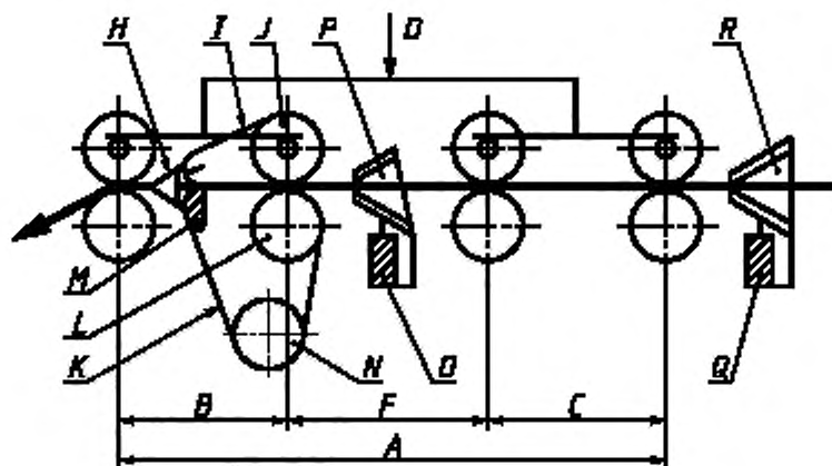
A — общая зона вытягивания; B — главная зона вытягивания; C — зона предварительного вытягивания; D — нагрузка на нажимные валики; F — зона уплотнения; H — передний уплотнитель; I — верхний ремешок; J — ведущий валик верхнего ремешка; K — нижний ремешок; L — цилиндр привода ремешков; M — направляющая нижнего ремешка; N — натяжное устройство нижнего ремешка; O — направляющая для крепления среднего уплотнителя; P — средний уплотнитель; Q — направляющая для крепления питающей воронки; R — питающая воронка
