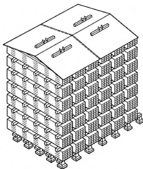
Рисунок А.6 — Пакетный штабель
