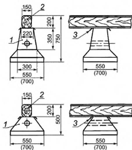
1 — опора, 2 — прогон, 3 — прокладка водонепроницаемая
