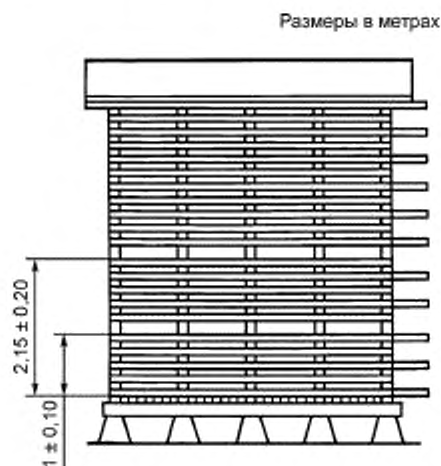
Рисунок А.9 — Горизонтальные каналы в рядовом штабеле
