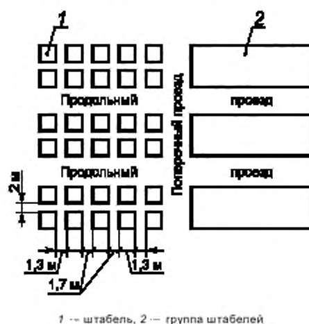
Рисунок А.1 — Планировка групп рядовых штабелей
