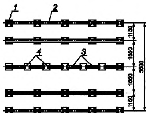
а) Укладка автопогрузчиком
