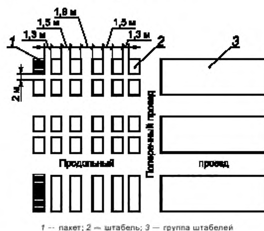
Рисунок А.2 — Планировка групп штабелей при пакетной укладке автопогрузчиком
