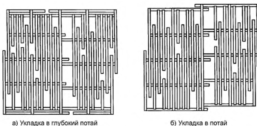
Рисунок А.8 — Способы укладки пиломатериалов в рядовые штабеля
