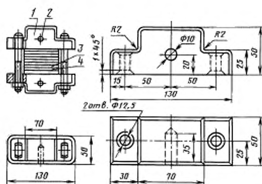
1 — обойма; 2 — отверстие для термометра; 3 — стальная прокладка; 4 — образец слюдяного материала
