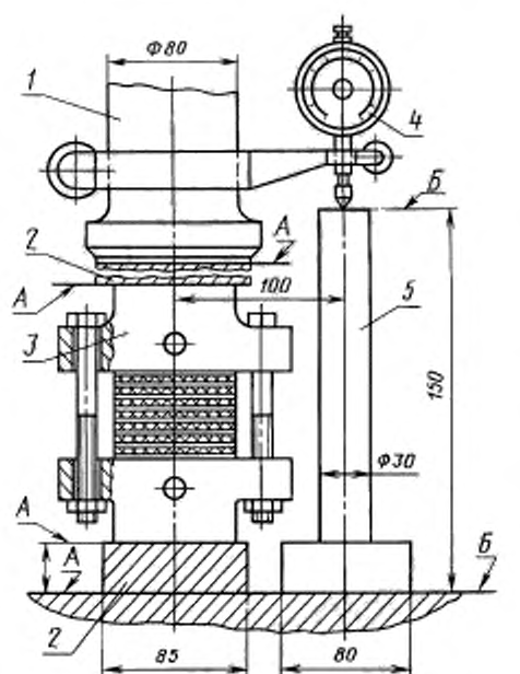
1 — шток; 2 — прокладка; 3 — оправка; 4 — индикатор часового типа; 5 — цилиндрическая подставка
