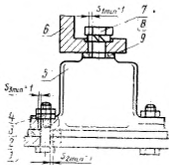
1—фундамент; 2—платин; 3—болт; 4—механизм; 5—амортизирующий элемент; 6—механизм; 7—винт; 8—шайба; 9—компенсирующий элемент
