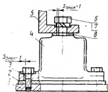
1—фундамент; 2—платин; 3—винт; 4—амортизирующий элемент; 5—механизм; 6—винт; 7—шайба; 8—компенсирующий элемент
