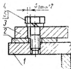
1—фундамент; 2—компенсирующий элемент; 3—механизм; 4—гайка; 5—шайба
