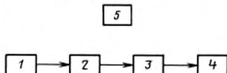
1 — лазер; 2 — ослабитель; 3 — оптическая система; 4 — устройство для измерения диаметра пучка излучения; 5 — средство юстировки
