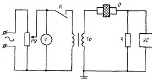
Тр—высоковольтный испытательный трансформатор; R—резистор; РУ—регулятор напряжения; О—образец с электродами; V—вольтметр для измерения напряжения пробоя; УС—устройство сигнализации о наступлении пробоя; К—контакт устройства сигнализации, отключающий первичную цепь трансформатора в момент пробоя образца
