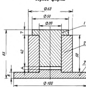
Пресс-форма
