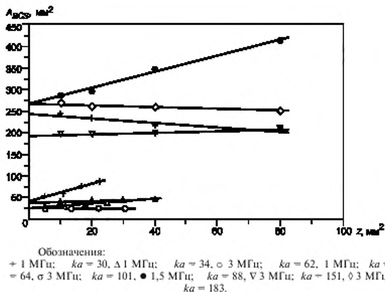
Рисунок И.1 — Зависимость площади поперечного сечения пучка от расстояния z до измерительной плоскости для восьми различных типов лечебных головок
