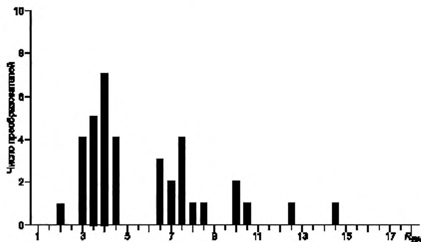
Рисунок В.2 — Гистограмма распределений значений R_{ax} для 37 лечебных головок различных диаметров и частоты
