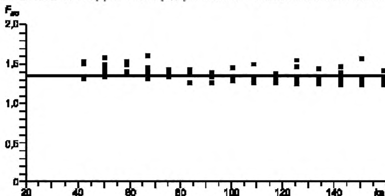
Рисунок Ж.1 — Зависимость коэффициента преобразования F_{ac} от ka для значений ka от 40 до 160
