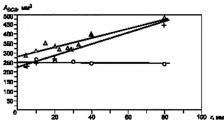
Рисунок И.2 — Зависимость площади поперечного сечения пучка от расстояния z до измерительной плоскости для трех излучателей с высокими R_{вз}
