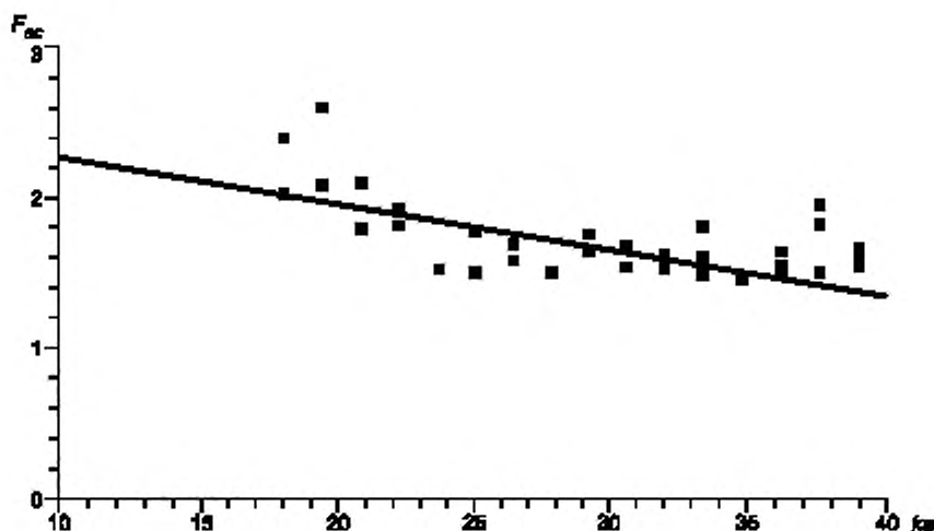
Рисунок Ж.2 — Зависимость коэффициента преобразования F_{ср} от ka для значений ka от 16 до 40
