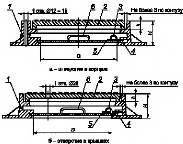
Рисунок А.8 — Люк ГТС с дополнительной крышкой
