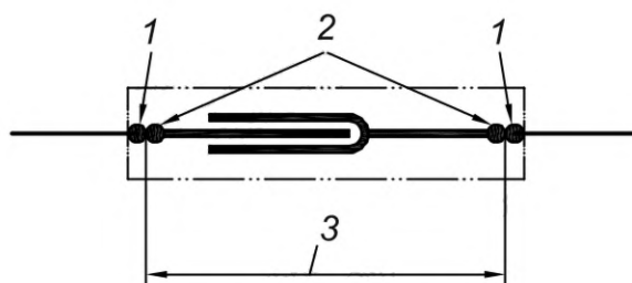
1 — точки измерения; 2 — присоединение проводника; 3 — контактное сопротивление
