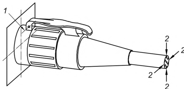
1 — шарнир крышки на розетке; 2 — усилие изгибающего момента
