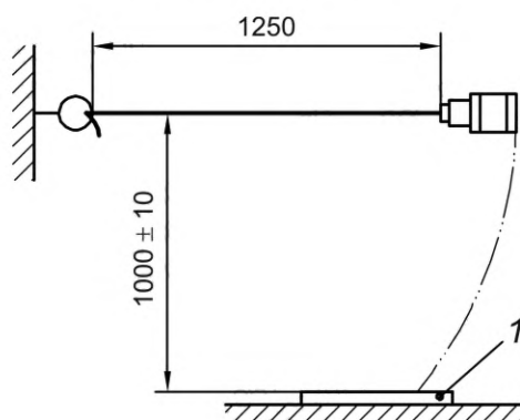
1 — стальная плита
