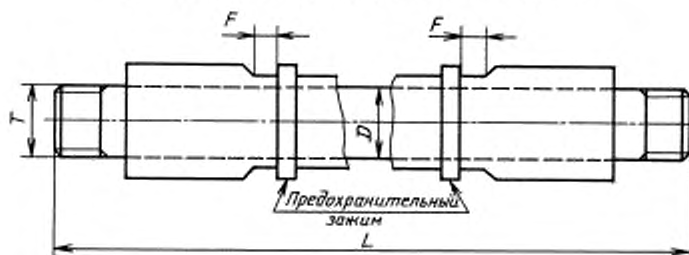
Размеры рукава бурового для гашения вибрации
