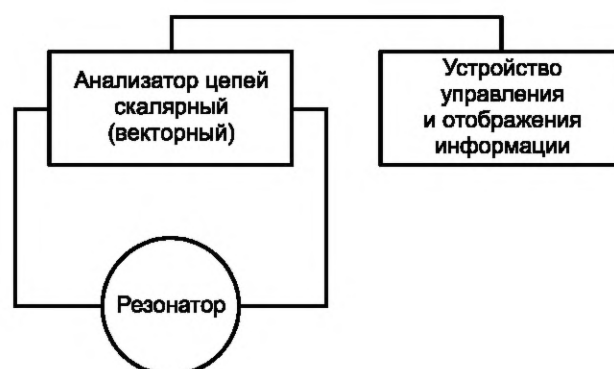
Рисунок 1 — Структурная схема измерительной установки для резонансных методов измерений \epsilon и \operatorname{tg} \delta
