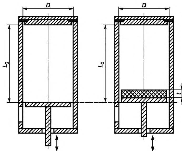
Рисунок А.3 — Схематическое изображение объемного резонатора с колебанием H_{01p} для измерений при фиксированной длине резонатора
