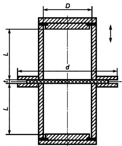
Рисунок А.4 — Схематическое изображение щелевого резонатора с колебанием H_{01p} для измерения подложек и листовых образцов
